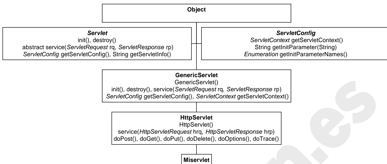
Figura 7. Jerarquía de clases en servlets.
