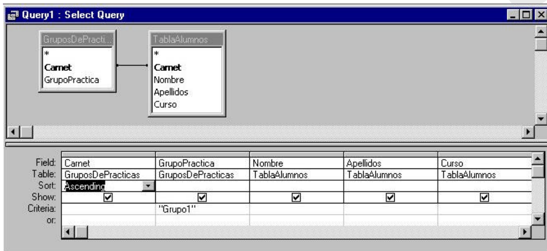
Figura 13. Relación entre campos de dos tablas.
